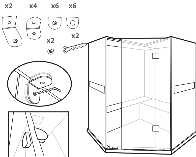
Paroi avant installée
