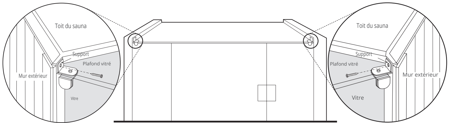
Paroi avant installée
